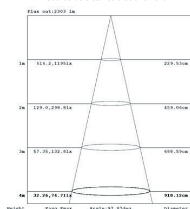
Courbe de distance d'éclairage
