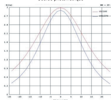
Courbe photométrique
