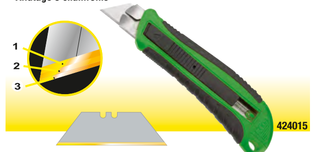
Affûtage 3 chanfreins
